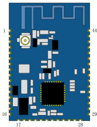
图 2 引脚标号
