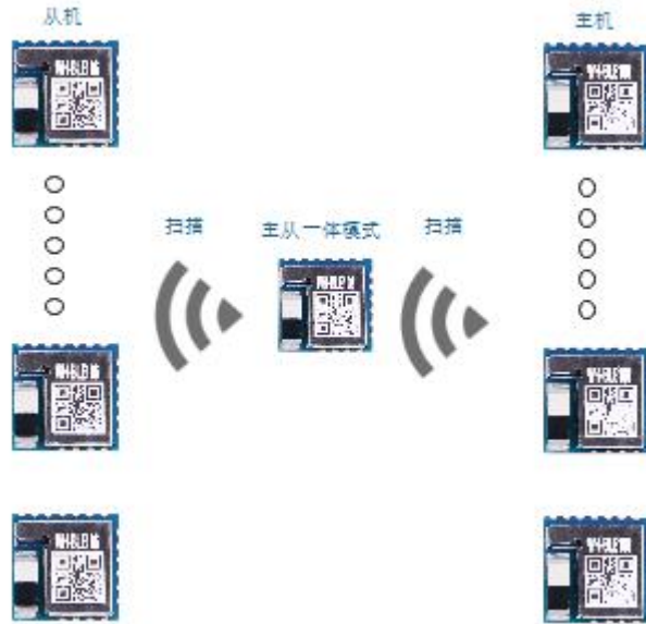
图 9 主从一体模式示意图
