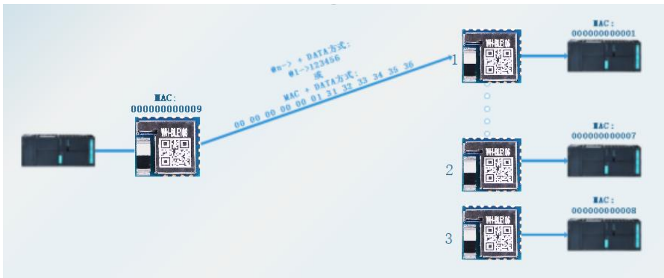
图 12 定点传输
