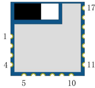
图 2 引脚标号
